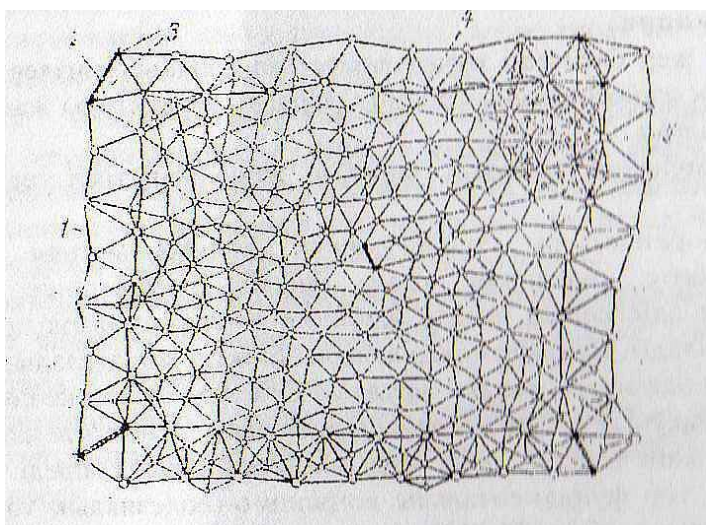
2-сурет. Мемлекеттік геодезиялық тор
