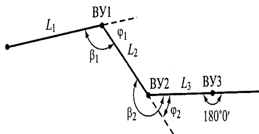
10 –сурет Трасса бойынша бұрылыстар бұрылуын анықтау
