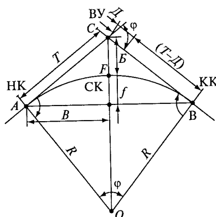
4-сурет. Қисық айналымының негізгі элементтері
